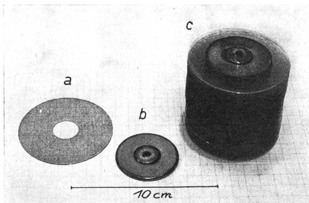
Fig. 6 Mehrfach-Plattenfunkenstrecke
