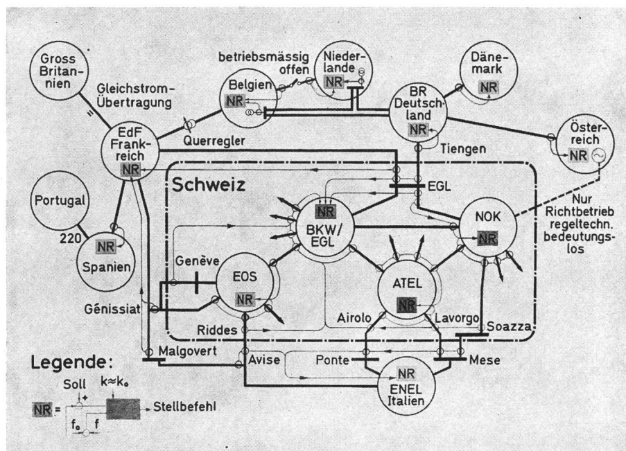
Fig. 3 Die schweizerischen Regelzentren und ihre Verbindungen mit den umliegenden Ländern
