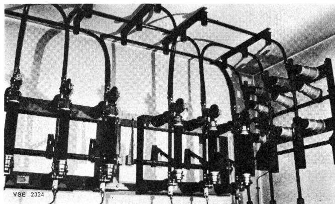
Fig. 8 PE-isolierte Hochspannungsleiter ohne Abschirmung in Transformatorenstation
