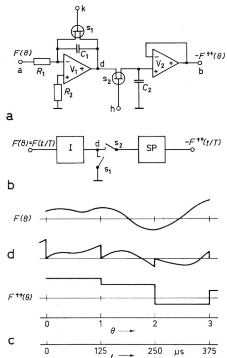
Fig. 5 Sequenztiefpas
