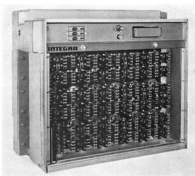
Fig. 4 Relaissatz für Weichensteuerung und Weichenverschluss
