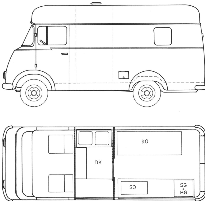
Fig. 2 Raumaufteilung im neuen Messwagen Maßstab \approx 1:50 DK Dunkelkammer; KO Kathodenstrahloszillograph; SO Schleifenoszillograph; SG Steuergerät; HG Hilfsgerät
