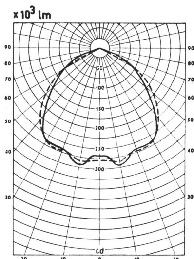
Fig. 3 Lichtstärkenverteilungskurve des Breitstrahlers von Fig. 2
