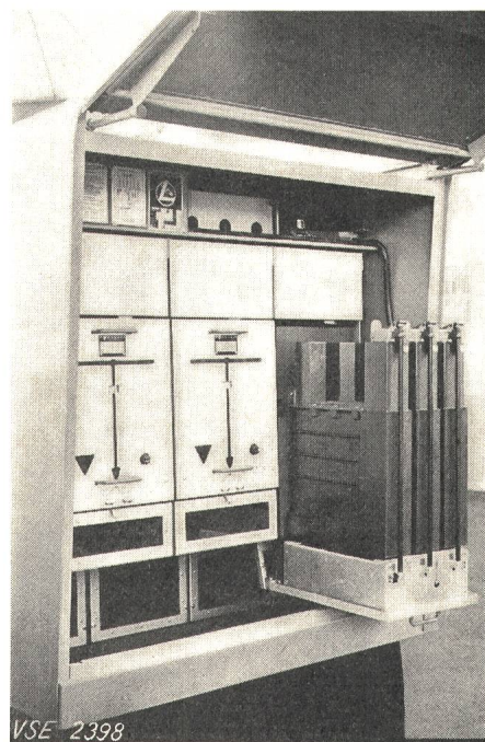
Fig. 5 Hochspannungsschaltschrank
