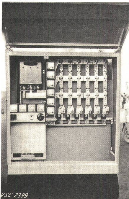
Fig. 6 Niederspannungsschaltschrank
