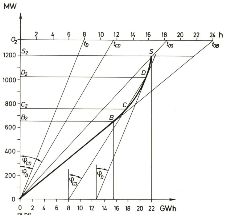
Fig. 5 Energieinhaltslinie des Verbrauches OS Energieinhaltslinie; O_2t_{OB} Ausnützungsstundenmaßstab
