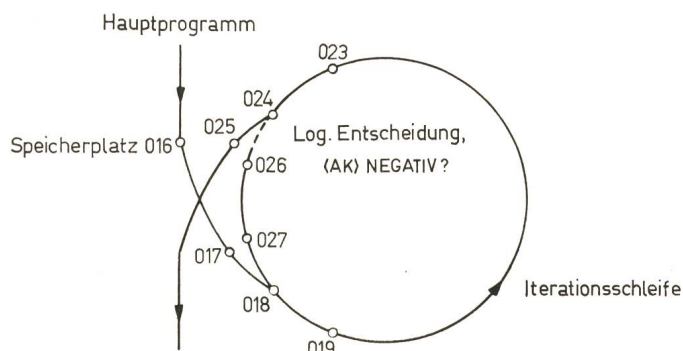
Fig. 7 Flussdiagramm des Programmablaufes
