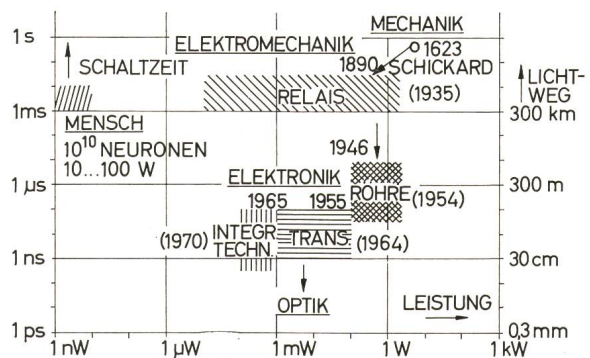
Fig. 13 Schaltzeit und Leistungsbedarf digitaler Schaltkreise
