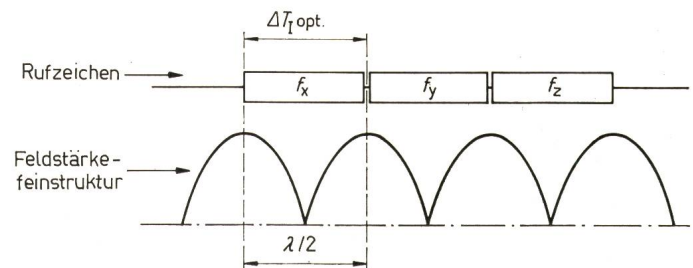
Fig. 3 Feldstärkeeinstruktur und optimale Impuls-Zeichenlänge \Delta T_{1 \text{ opt.}} optimale Impulslänge; f_x, f_y, f_z Codefrequenzen; \lambda HF-Wellenlänge
