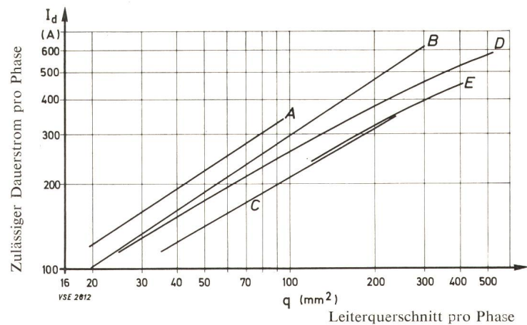
Fig. 6 16 kV-Freileitungen
