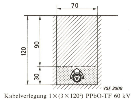
Fig. 4 Kabelverlegungsarten
