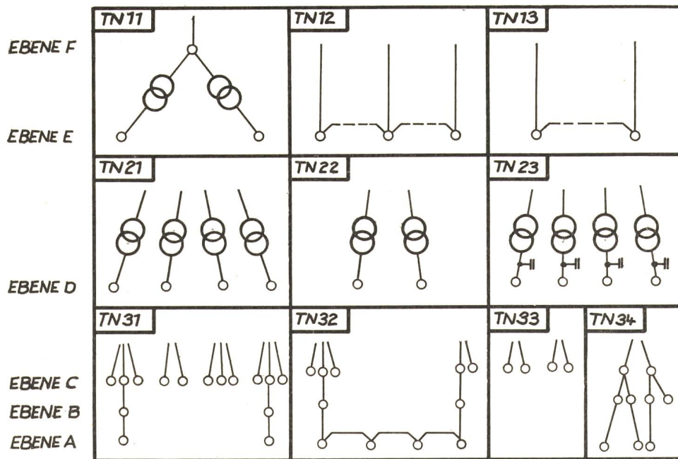
Fig. 4 Prinzipdarstellung zum Aufbau eines Netz- schemas aus Teilnetzen
