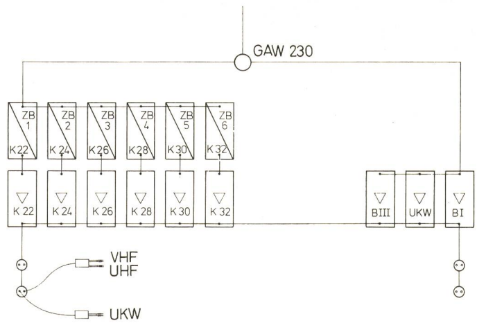
Fig. 14 Verteilverstärker mit Bereichsverstärkern für die Bänder I—III und Umsetzern für den Zwischenbereich
