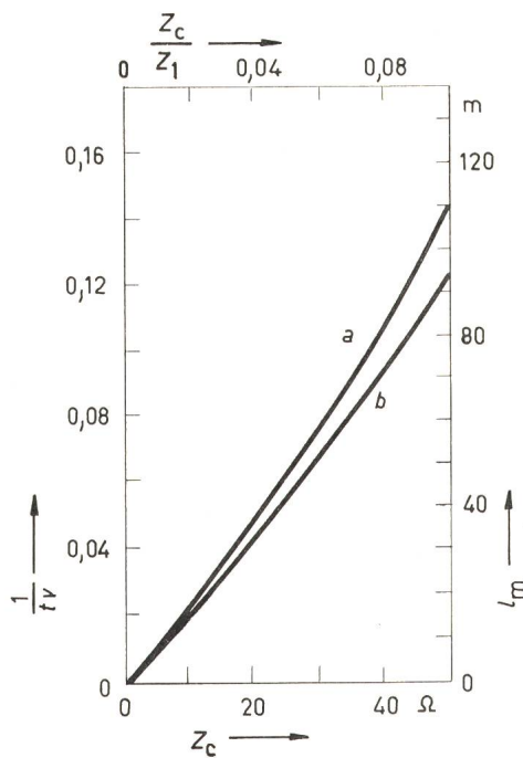
Fig. 1 Selbstschützende Kabellängen
