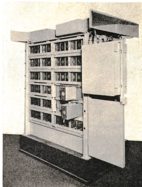
Fig. 11 Stromrichterblock für die beiden parallelgeschalteten Fahrmotoren eines Drehgestells einer Re 4/4 Anschluss-Wechselspannung: 2 \times 738 V Stundenstrom: 2600 A
