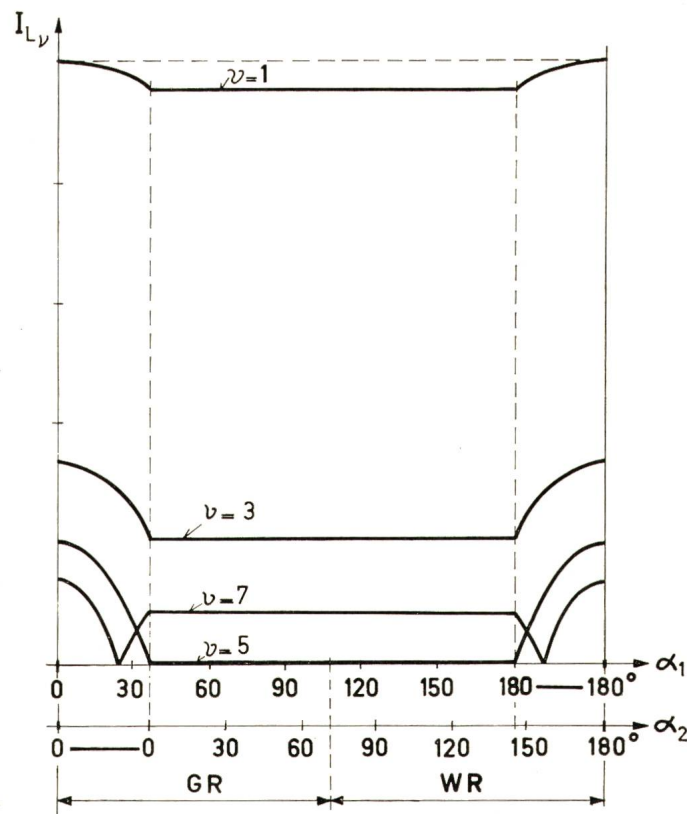
Fig. 9 Oberwellenamplituden des simultan folgesteuerten Stromrichters in Funktion der Ansnittwinkel Bezeichnungen siehe Fig. 7
