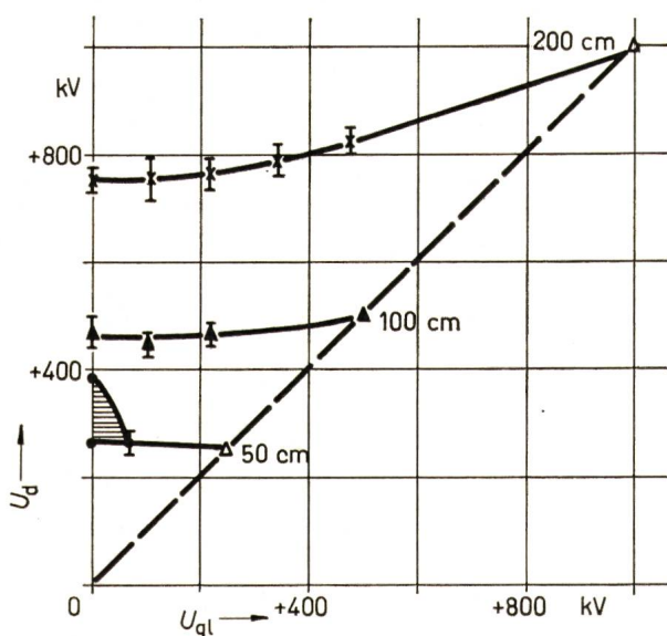
Fig. 10 Durchschlagspannung von Stab-Platte-Funkenstrecken bei Überlagerung von Gleich- und Stoßspannung 60/525 \varphi_a \approx 7...11 \text{ g/m}^3 ; Parameter: Elektrodenabstand Bezeichnungen siehe Fig. 4
