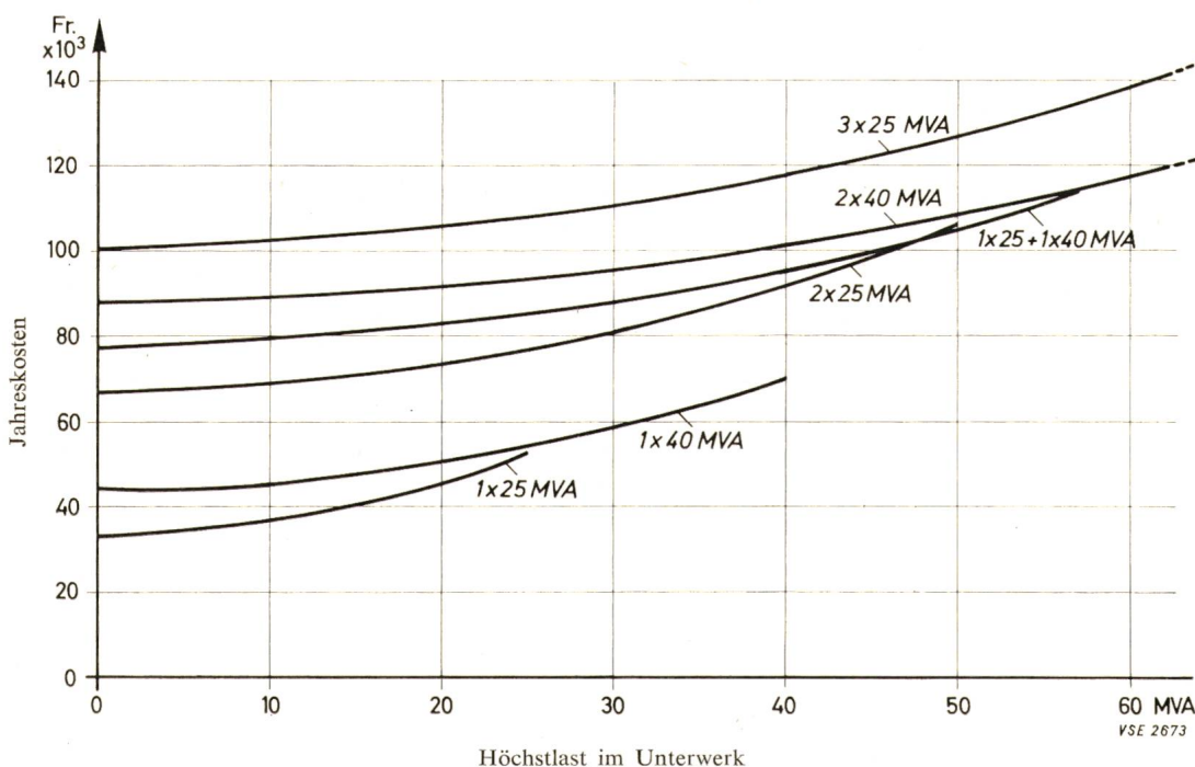
Fig. 7 Jahreskosten von 50/16-kV-Reguliert-Transformatoren (bei einer Gebrauchsdauer der Höchstlast von 4700 Stunden pro Jahr)
