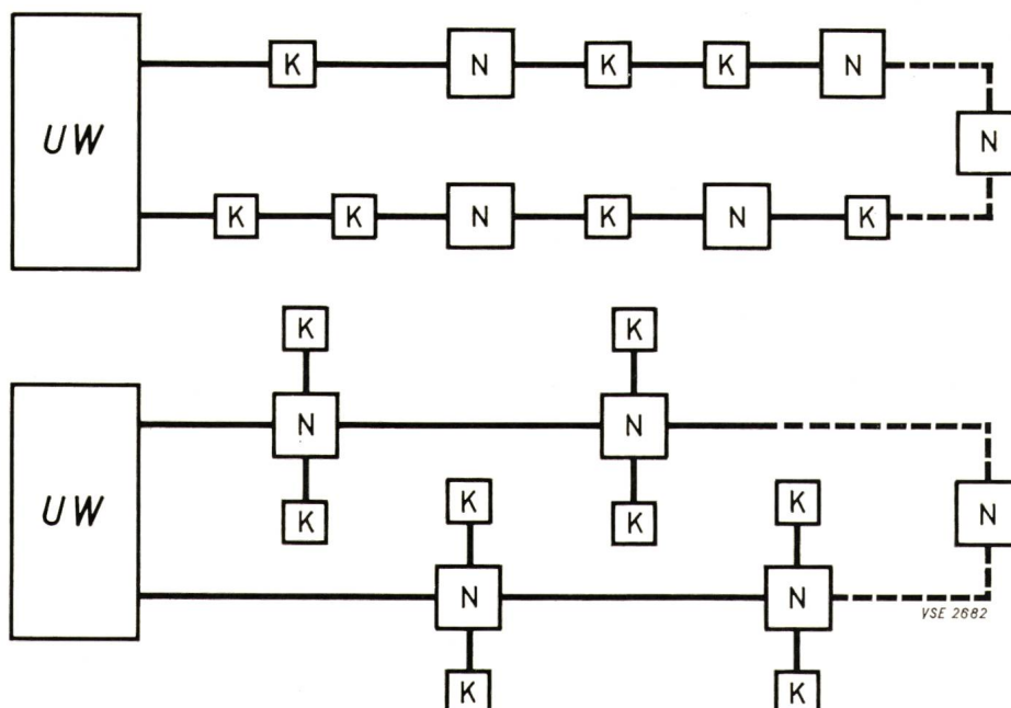
Fig. 15 Möglichkeiten für einen Netzausbau mit Kompaktstationen UW = Unterwerk N = Normalstation K = Kompaktstation
