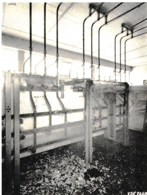
Fig. 2 Wirkung eines Kurzschlusses ohne Sammelschienenschutz
