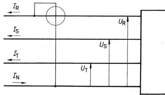
Fig. 3 Kunstschtaltung des Leistungsmessers für die Messung der Wirkleistung Bezeichnungen siehe Fig. 2
