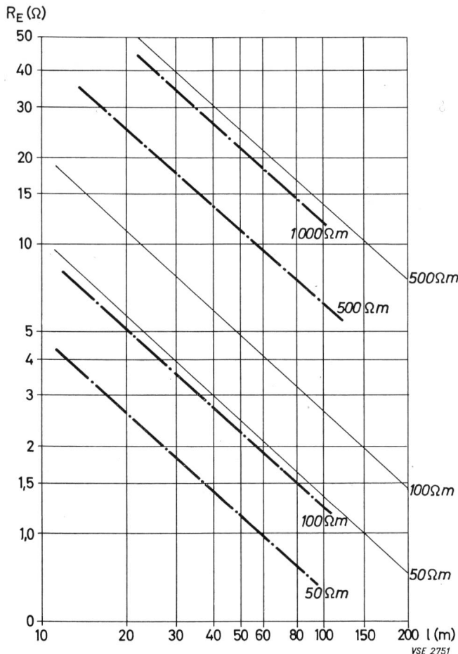
Fig. 1 Ausbreitungswiderstand von gestreckten Bändern von Tieferdnern (2 cm \phi )
