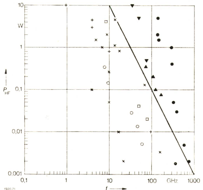
1920 71 Fig. 1 Dauerstrichleistung P_{HF} von Röhren- und Halbleiteroszillatoren als Funktion der Frequenz f ○ Gunndiode □ LSA-Diode × Lawinendiode + Vervielfacherdiode ▲ Reflexklystron ▼ Doppelspaltoszillator ● Rückwärtswellenröhre — Leistungsgrenze zwischen Röhren- und Halbleiteroszillatoren im Bereich 10 GHz bis 1000 GHz
