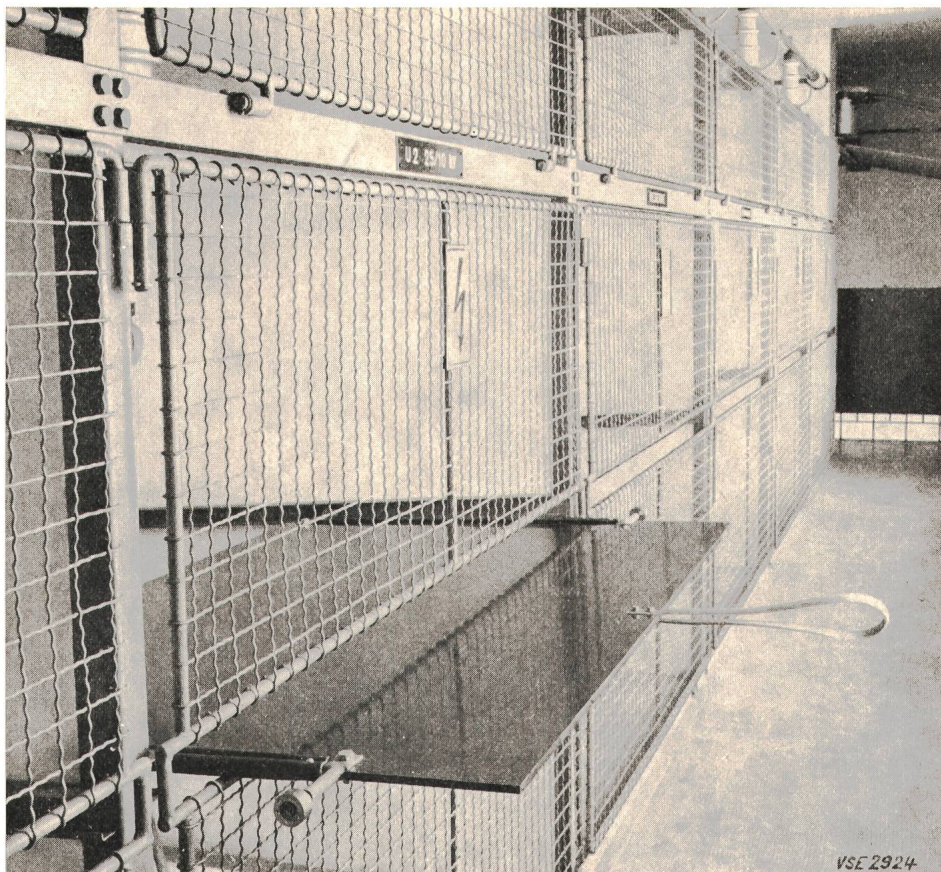
Fig. 1 Einschub-Schutzplatte (mit Bedienungsschleufe) in einer 25 kV-Schaltanlage (OKA) Ein gefahrloses Einschieben der Platte bereits vor dem Öffnen des Gitters wird durch einen Schlitz in letzterem erreicht.
