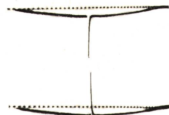
Fig. 5 Negativer Normstoss im negativen Scheitel der Wechselspannung Schaltung gemäss Fig. 1a
