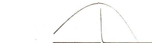
Fig. 7 Positiver Normstoss im positiven Scheitel der Wechselspannung Schaltung gemäss Fig. 1b
