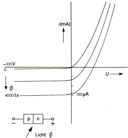
Fig. 19 Kennlinienfeld der Photodiode U Spannung an der Diode i Strom durch die Diode
