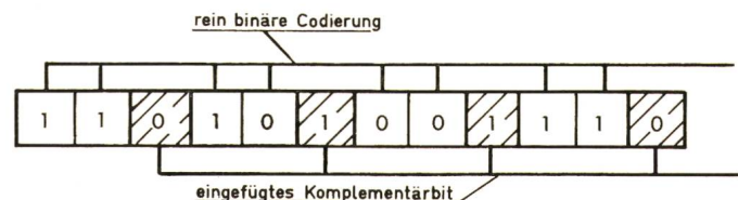
Fig. 2 Rein binäre Codierung mit eingefügtem Komplementärbit
