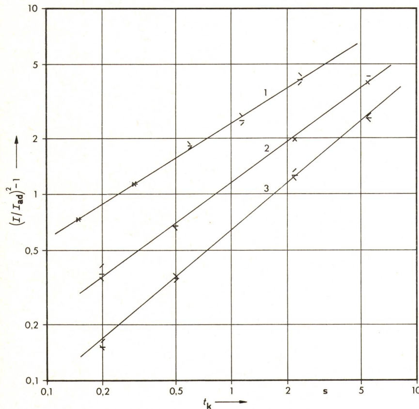
Fig. 3 Relative Belastbarkeit (I/I_{ad})^2 - 1 der Schirme der Kabel 1, 2 und 3, abhängig von der Kurzschlusszeit t_k für die Kurzschlusswärmerhöhung \vartheta_k - 20 K der Schirme von 50, 100 und 200 K
