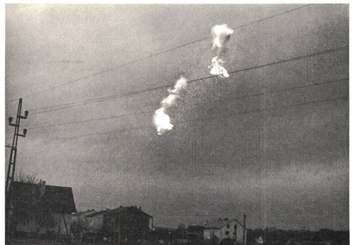
Fig. 5 Lichtwirkungen eines über eine Metallitze eingeleiteten, frei brennenden Kurzschluss-Lichtbogens gemäss Fig. 4; nach einer Zeit von 440 ms bereits weitgehend abgeebbt.
