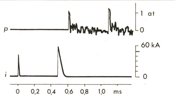
Fig. 4 Oszillogramm der Druckwellen ( p ), gemessen in 30 cm Abstand vom Blitzkanal, in dem zwei Stromstösse ( i ) fliessen Laufzeit der Druckwellen bis zur Meßstelle, 0,6 ms
