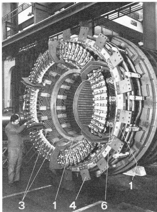
Fig. 4 Stator eines grossen Generators Bezeichnung siehe Fig. 5
