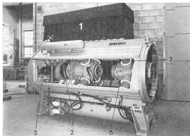
Fig. 9 Druckluft Generatorschalter
