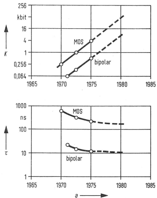
Fig. 1 Kapazität K und Zugriffszeit \tau von MOS- und Bipolarbausteinen in bezug auf das Herstellungsjahr.
