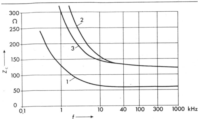
Fig. 3 Impédance caractéristique Z_c en fonction de la fréquence f
