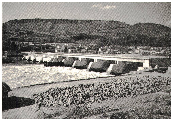
Fig. 4 Niederdruck-Laufkraftwerk Rheinkraftwerk Säkingen AG (Partnergesellschaft). Stauwehr im Vordergrund und anschliessendes Maschinenhaus.
