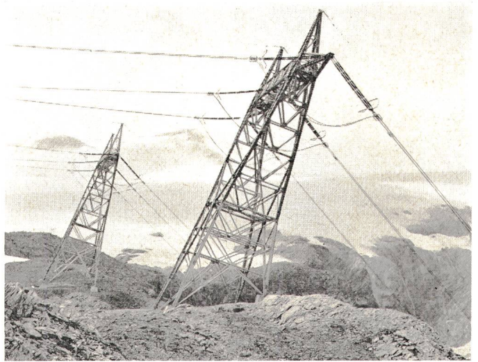
Fig. 7 380-kV-Freileitung Tavanasa–Breite. Abspannmasten am Vorab-Gletscher, 2610 m ü. M.
