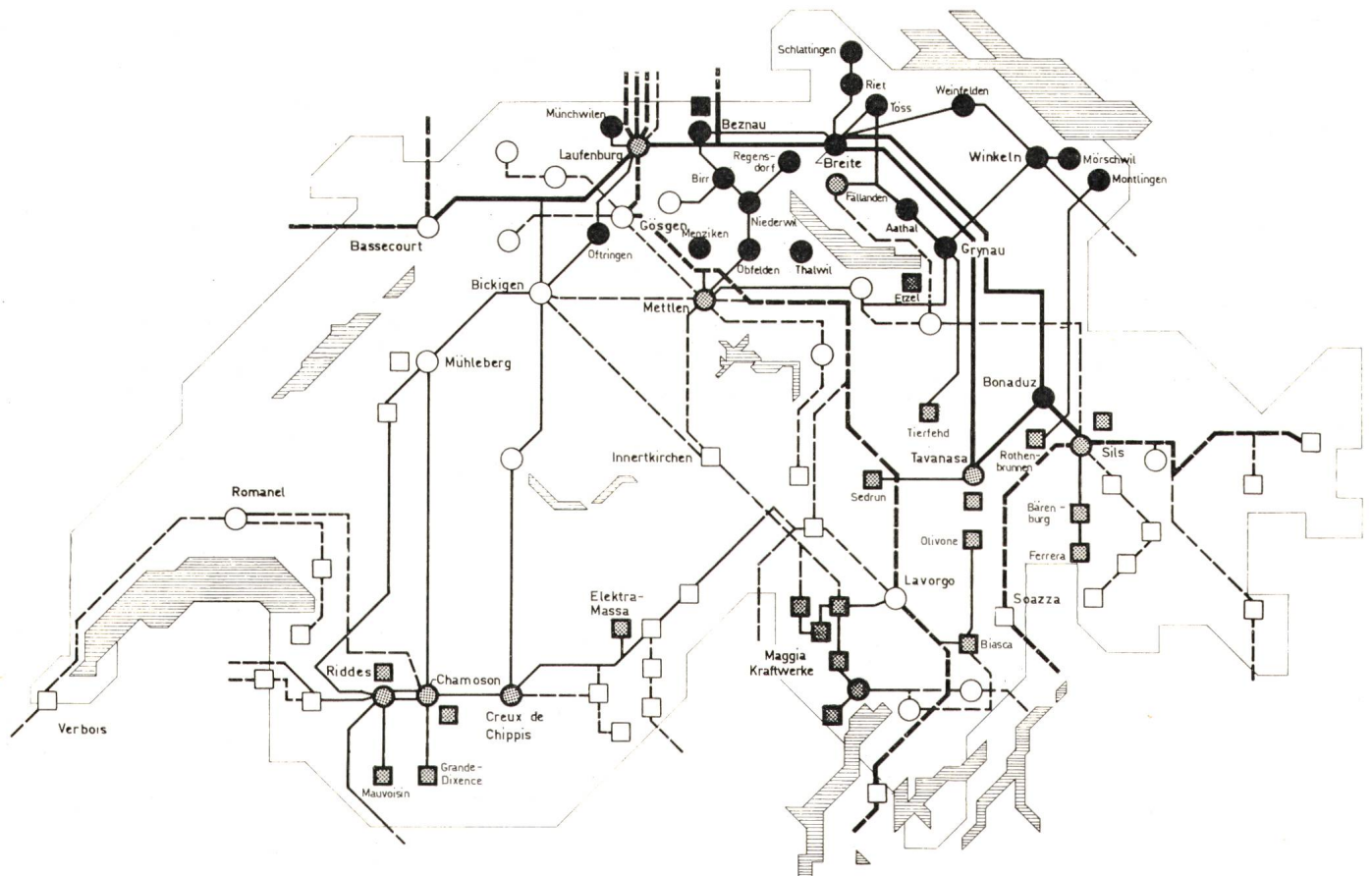
Fig. 8 380/220-kV-Höchstspannungsnetz
