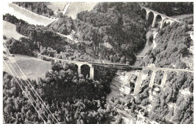
Fig. 3 Kraftwerk Kubel mit Stausee und altem Zentralengebäude Im Hintergrund ist die Zufahrtsbrücke zur neuen Kavernen-Zentrale, in der Mitte das Viadukt der Bodensee-Toggenburg-Bahn und im Vordergrund die 220-kV-Leitung der NOK über das Sittertobel ersichtlich.
