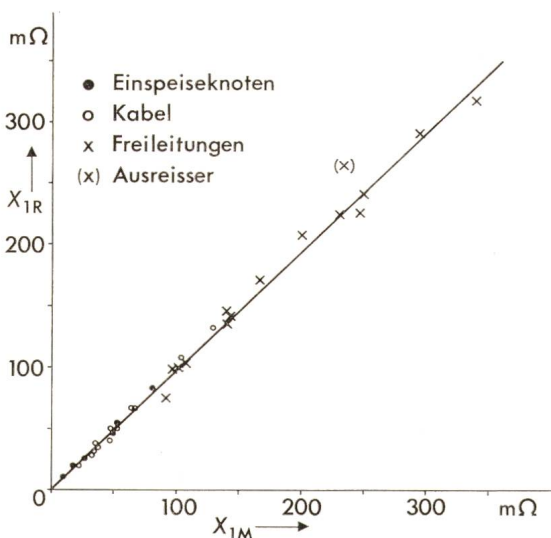
Fig. 3 Berechnete Reaktanz X_{1R} des Mitsystems in Abhängigkeit von der gemessenen Reaktanz X_{1M}
