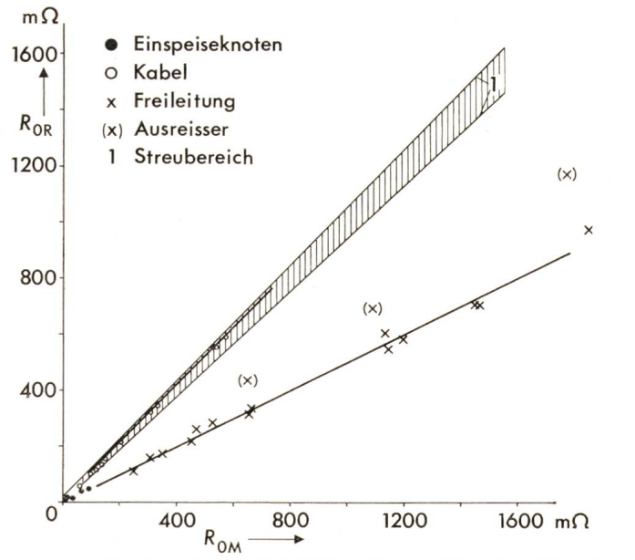
Fig. 4 Berechnete Resistanz R_{0R} des Nullsystems in Abhängigkeit von der gemessenen Resistanz R_{0M} [1]
