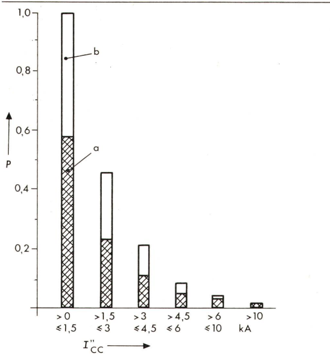
Fig. 2 Wahrscheinlichkeit P des Auftretens von Kurzschluss-Strömen I'' CC einer bestimmten Grössenklasse im Fall eines Kurzschlusses an den Eingangsklemmen der Leitungsschutzschalter oder Sicherungen a) gültig für Ströme innerhalb des angegebenen Bereiches b) gültig für Ströme oberhalb des angegebenen Bereiches
