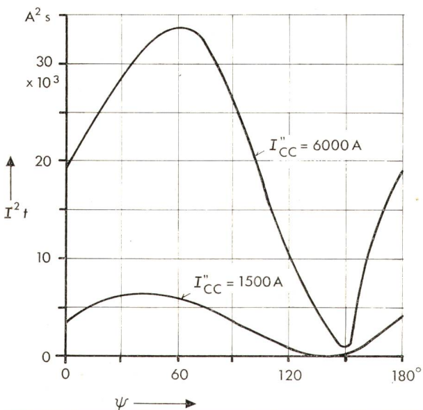
Fig. 6 Empirisch ermittelte I^2t -Mittelwerte, als Funktion des Draufschaftwinkels \psi , bei U_t = 250 \text{ V} , \cos\phi = 0,9 und U_{\text{arc}} = 300 \text{ V}
