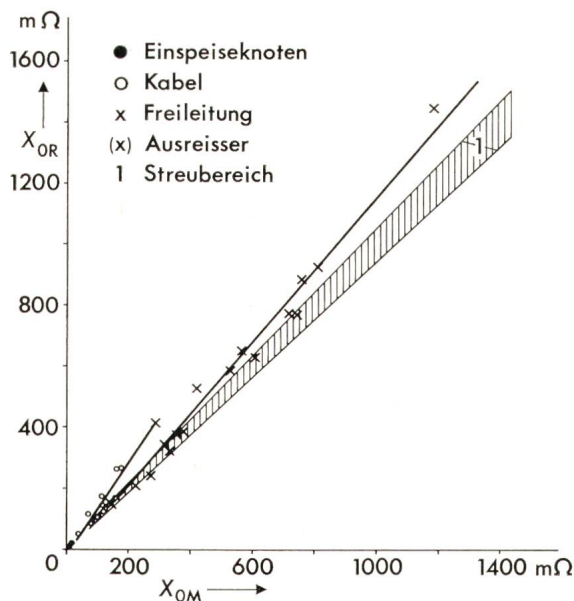
Fig. 5 Berechnete Reaktanz X_{OR} des Nullsystems in Abhängigkeit von der gemessenen Reaktanz X_{OM} [I] Ausgleichsgerade [mΩ] X_{OR} = -14,96 + 1,495 X_{OM} (Kabel) X_{OR} = -31,69 + 1,184 X_{OM} (Freileitung)
