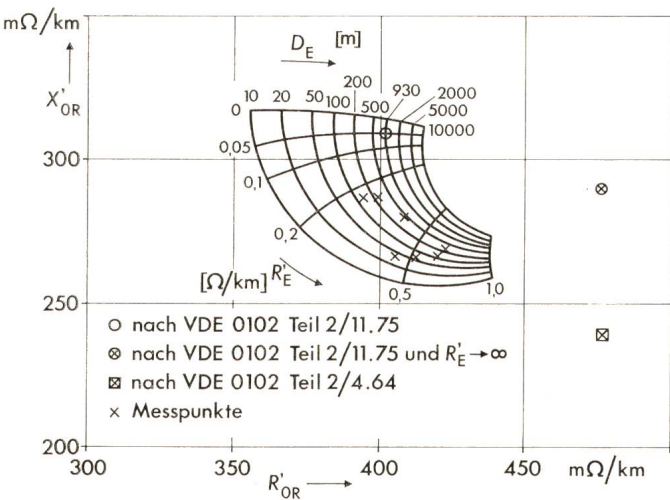
Fig. 1 Berechneter Reaktanzbelag X'_{OR} des Nullsystems für Kabel TT 4 \times 240 \text{ mm}^2 Al(se) in Abhängigkeit vom berechneten Resistanzbelag R'_{OR} des Nullsystems
