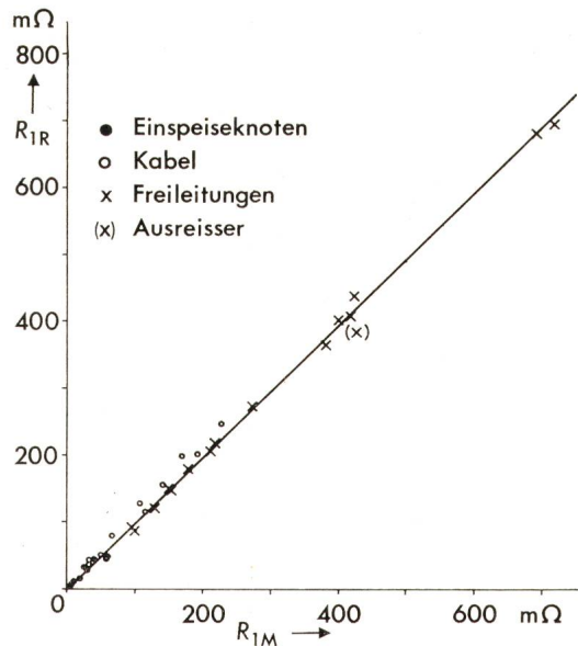
Fig. 2 Berechnete Resistanz R_{1R} des Mitsystems in Abhängigkeit von der gemessenen Resistanz R_{1M}
