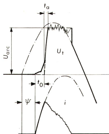
Fig. 3 Strom- und Spannungsverlauf eines strombegrenzenden LS-Schalters beim Abschalten eines Kurzschlusses - - - - - eingeschwungener Zustand - - - - - für die Rechnung angenommener Verlauf der Lichtbogen-Spannung ψ Draufschaftwinkel (Moment des Entstehens des Kurzschlusses) t 0 Öffnungszeit t a Ausbildungszeit des Lichtbogens U arc Lichtbogen-Spannung
