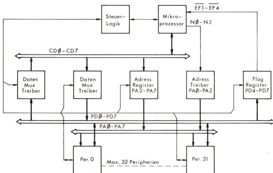
Fig. 4 Peripherie-Bussystem CD \emptyset -CD 7 Mikroprozessor Datenbus PD \emptyset -PD 7 Peripherie Datenbus PA \emptyset -PA 7 Peripherie Adressbus N \emptyset -N 2 Ein-/Ausgabe-Befehlssignale \overline{\text{EF}}1 - \overline{\text{EF}}4 Peripheriestatus Eingänge
