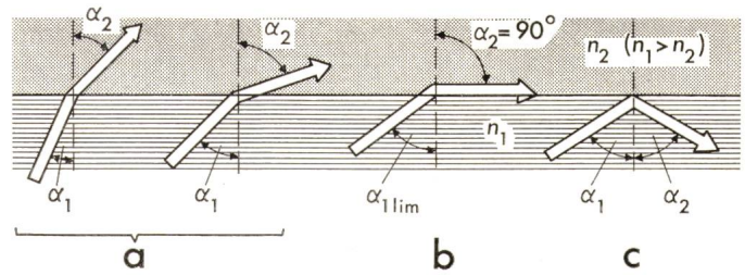
Fig. 1 Comportement d'un rayon lumineux à l'interface de deux milieux transparents d'indices n_1 et n_2
