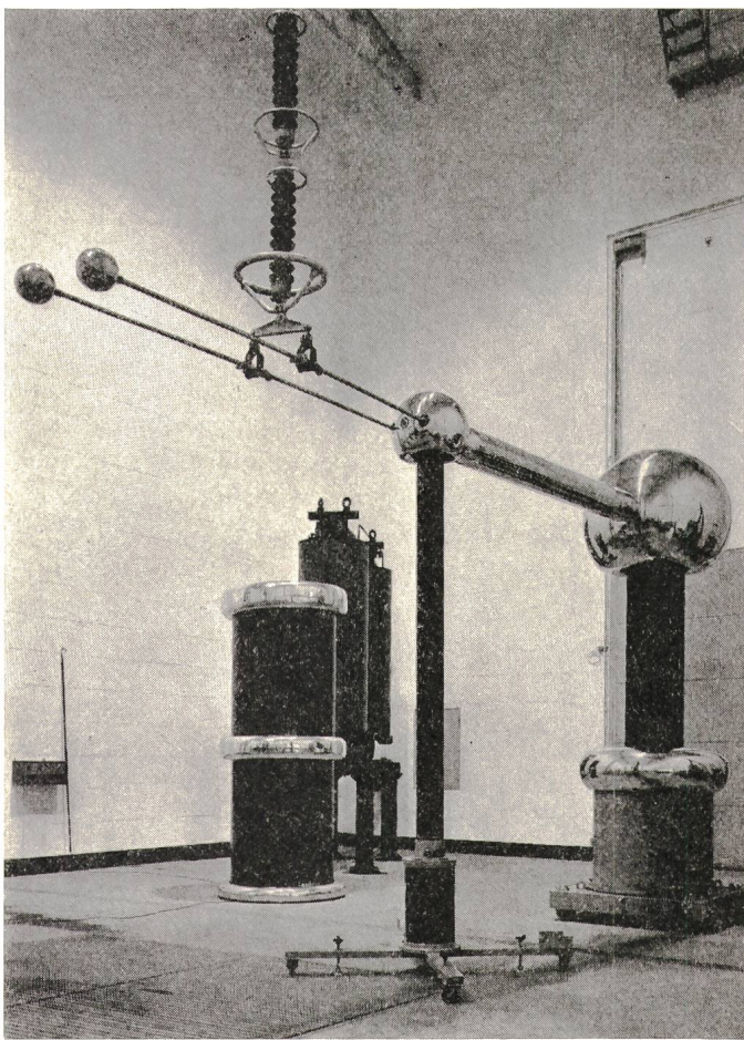
Fig. 5 Radiostörfreier Transformator für Teilentladungsmessungen bis 300 kV mit angeschlossenen Kopplungskondensator (2000 pF) Geprüft werden im Bild die Armaturen einer Freileitungsisolatorenkette (Leiteraufhängung mit Joch und Schutzringen).
