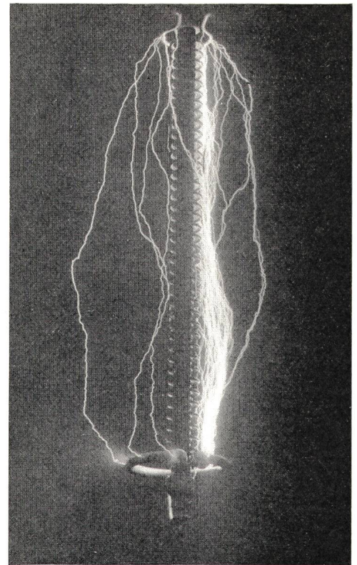
Fig. 6 Überschlag bei einer Wechselspannung von ca. 1 MV
