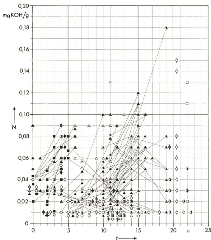
Fig. 4 Neutralisationszahl N in Abhängigkeit der Anzahl Betriebsjahre \alpha Erklärung der Symbole in Tabelle III
