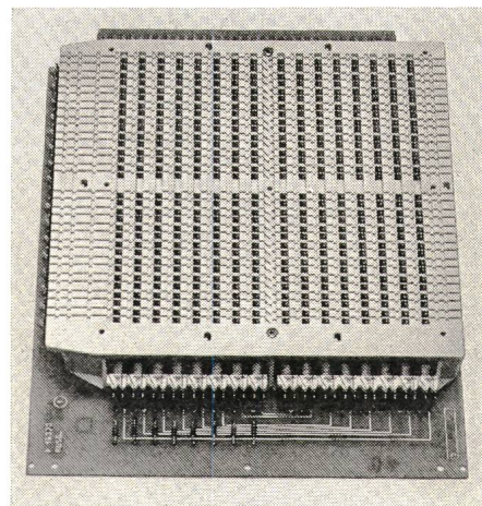
Minikreuzschalter
