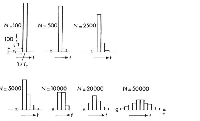
Fig. 9 Impulsantwort einer N -stufigen Verzögerungskette \varepsilon = 10^{-4} Verlustfaktor f_T Taktfrequenz
