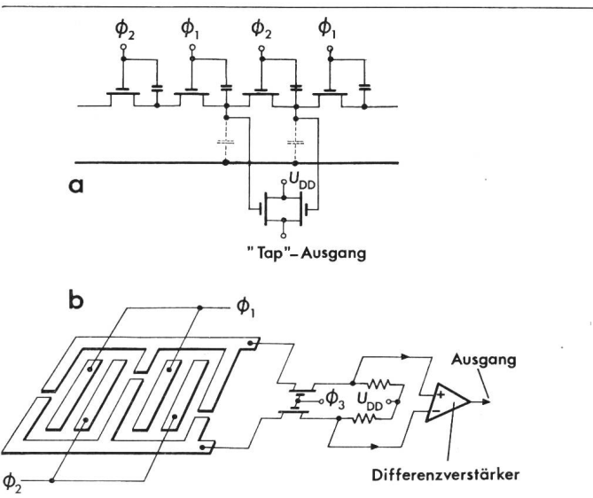
Fig. 8 a) Anzapfschaltung (Tap) an einer BBD-Verzögerungsleitung und b) Split-Elektroden Version der Floating-Gate-Technik für die Anzapfung von CCD-Zellen (dreiphasige CCD-Speicherzellen). Die auf den geteilten Elektroden in b) influenzierte Ladung wird differentiell gemessen und addiert bei gleichzeitiger Speisung aus \Phi_3 [6]
