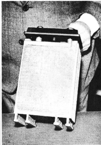
Fig. 6 Blei-Kobalt-Batterie, die im Personenfahzeug «Transformer I» (Fig. 11) serienmässig eingebaut ist
