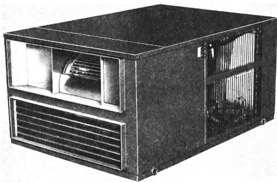
Fig. 1 Pompe à chaleur air-air type monobloc
