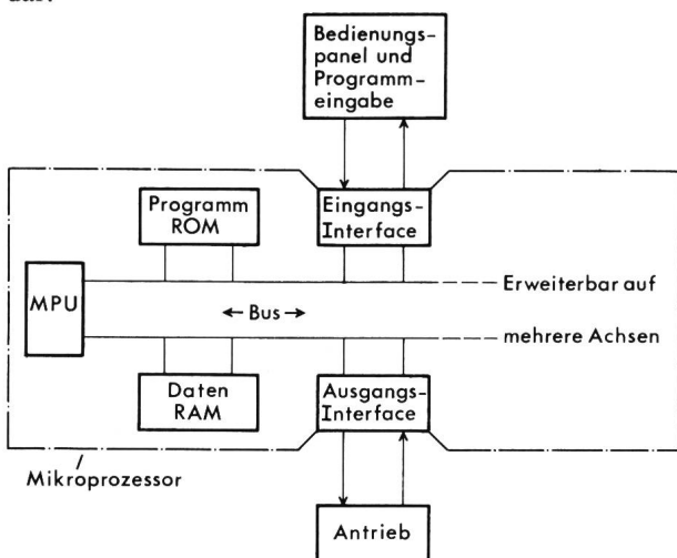
Fig. 1 Aufbau einer Positioniersteuerung mit Mikroprozessor MPU Microprocessor Unit RAM Random Access Memory ROM Read Only Memory
