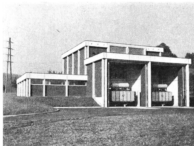
Fig. 9 Unterstation Willisau
