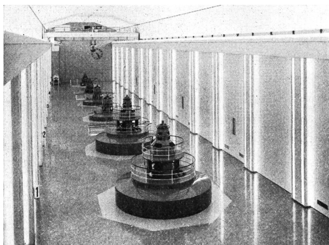
Fig. 5 Maschinsaal mit Generatoren des Kraftwerkes Göschenen
