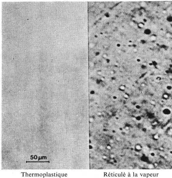
Fig. 9 Polyéthylène sans et avec des microvoids
