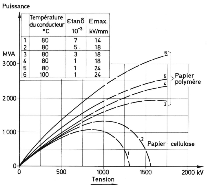
Fig. 6 Puissance de transport de câbles à huile de 1200 mm 2 (selon Fujita)
