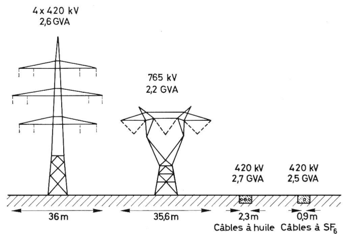
Fig. 4 Largeurs des cheminements pour les divers systèmes de transport (selon Eidinger et Klement)
