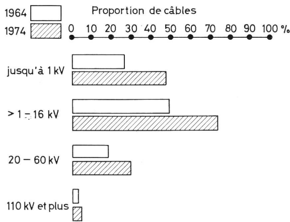
Fig. 3 Proportion de câbles par rapport à la longueur totale des lignes en Allemagne (selon VDEW)
