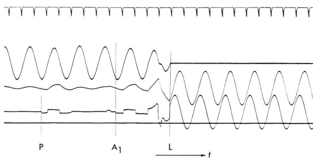
Fig. 5 Oszillogramm einer Trennerkommutierung mit kurzer Prell- und Löschzeit
