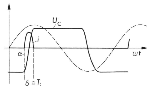
Fig. 6 Einpulsiger Stromrichter mit LC-Last: Schaltung und Oszillogramme
