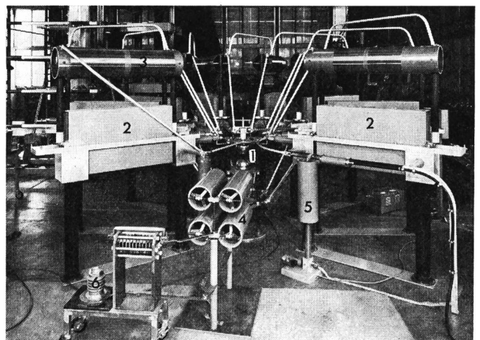
Fig. 13 Kombierter Stoßstromgenerator 100 kV, 80 kJ für Hochstromimpuls 4/10 \mu\text{s} , 200 kA und Langzeitstoss 2100 \mu\text{s} , 700 A
