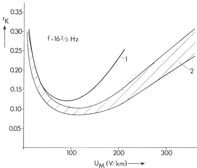
Fig. 6 Reduktionsfaktoren in Abhängigkeit von der induzierten Spannung in der Kabelhülle bei f = 16\frac{2}{3} Hz für die 56''-Streckenfernmeldekanal der BLS
