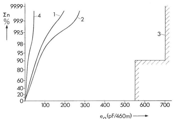
Fig. 8 Erdkopplungen der 56''-Streckenfernmeldekanal der BLS für Werkklängen und für ausgeglichene Spulenfelder
