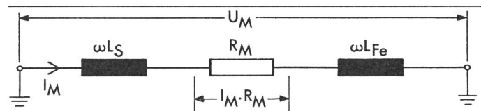
Fig. 3 Ersatzschaltbild einer Kabelhülle mit metallischem Kabelmantel und Bewehrung aus Bandeisern
