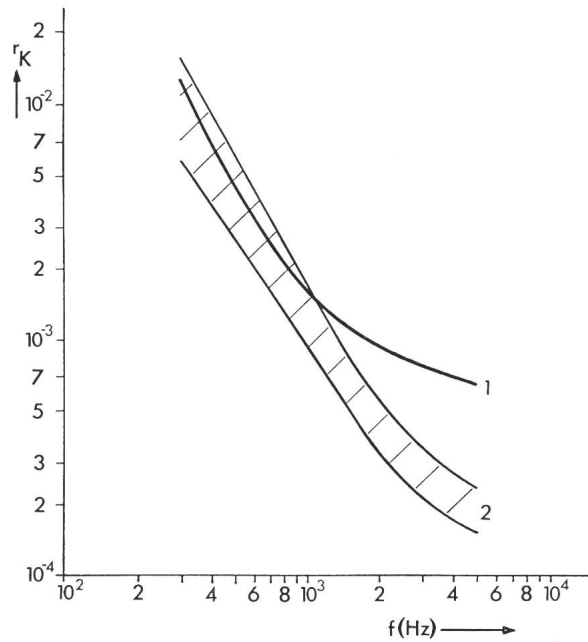
Fig. 7 Reduktionsfaktoren in Abhängigkeit von der Frequenz für die 56''-Streckenfernmeldekanal der BLS
